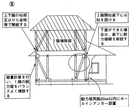
2階を増築した場合の1階耐力壁増設
